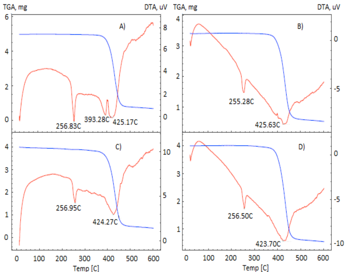
Рисунок 4.8. Кривые ТГА (синяя) и ДТА (красная): полубархатная ткань (А), полубархат-ПМА (В), велюровый трикотаж (С) и «велюровый трикотаж-ПМА» (D)
