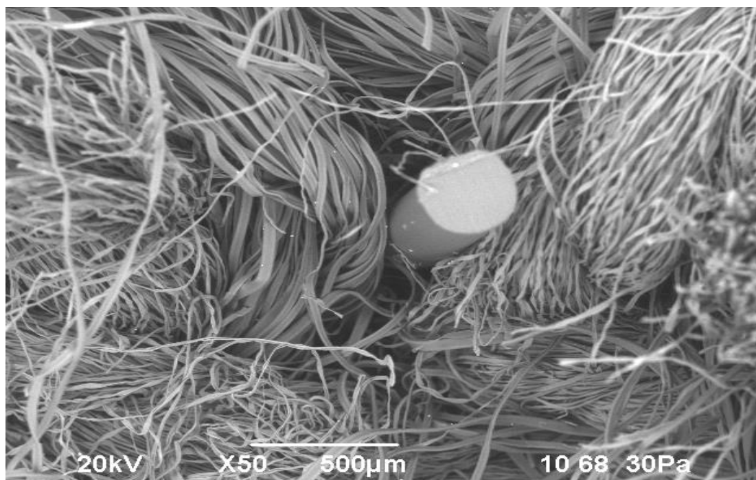
Рисунок 3.9 - Морфология поперечного сечения трикотажного полотна с полимерным оптическим волокном.
