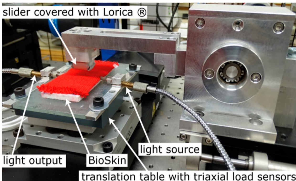
Рисунок 2.2 Установка для испытаний на трение и сжатие.
