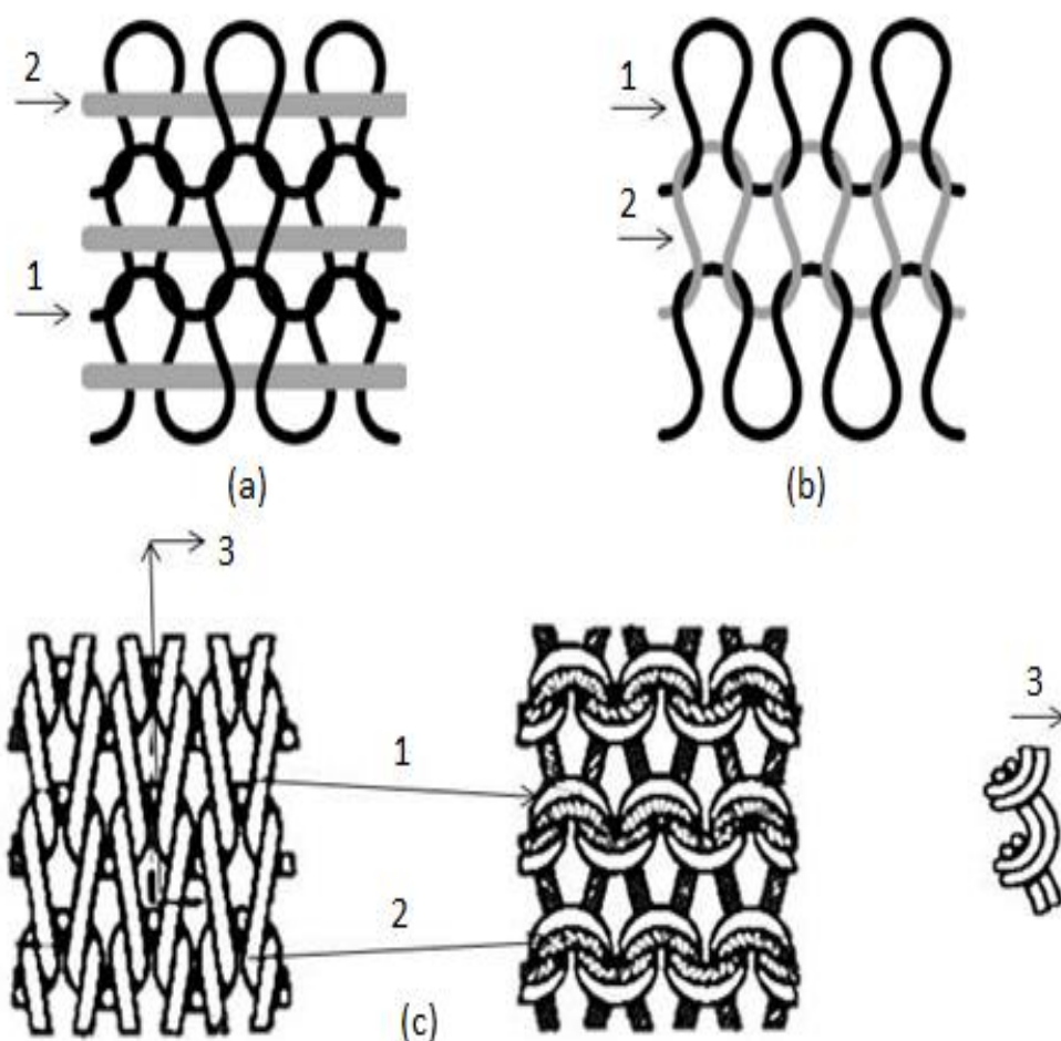
Рисунок 2.1 - Примеры вязаной структуры: (a) простое переплетение с оптическим волокном в качестве уточной нити (1 - хлопковая пряжа, 2 - оптическое волокно); (b) оптическое волокно участвует в простом переплетении (1 - хлопковая пряжа, 2 - оптическое волокно); (c) оптическое волокно участвует в плюшевом переплетении (1 - оптическое волокно, 2 - хлопковая пряжа, 3 - плюшевый узел)
