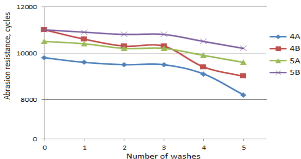
Рисунок 4.15 - Зависимость устойчивости к истиранию образцов полимерно-текстильных материалов №4 и №5 от числа стирок
