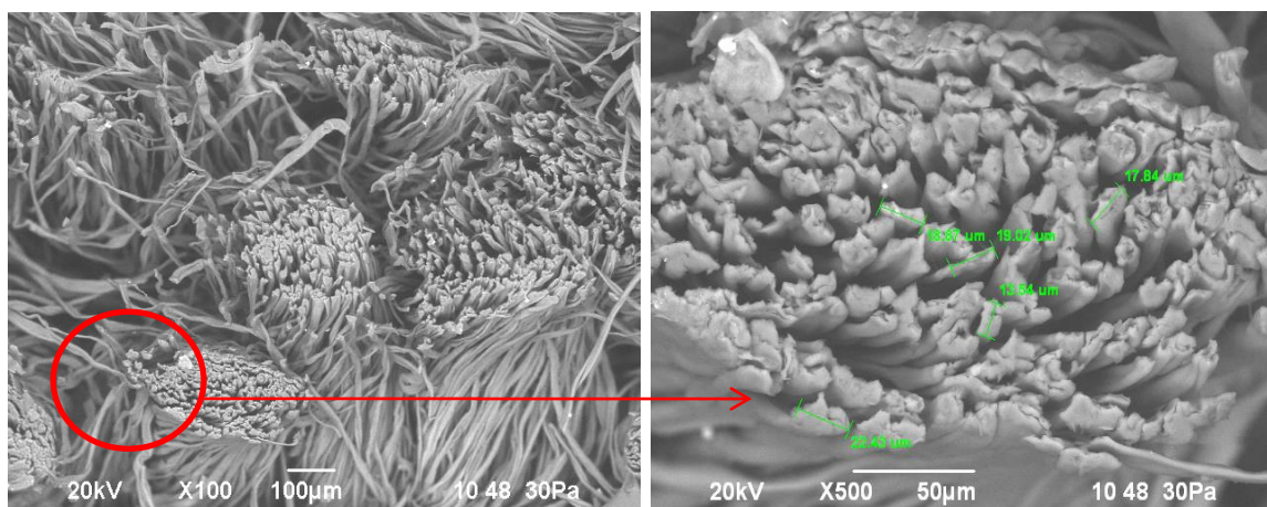
Рисунок 4.11 - СЭМ изображения поперечного среза махровой хлопковой ткани до нанесения (сверху) и после нанесения акриловой эмульсии (снизу)
