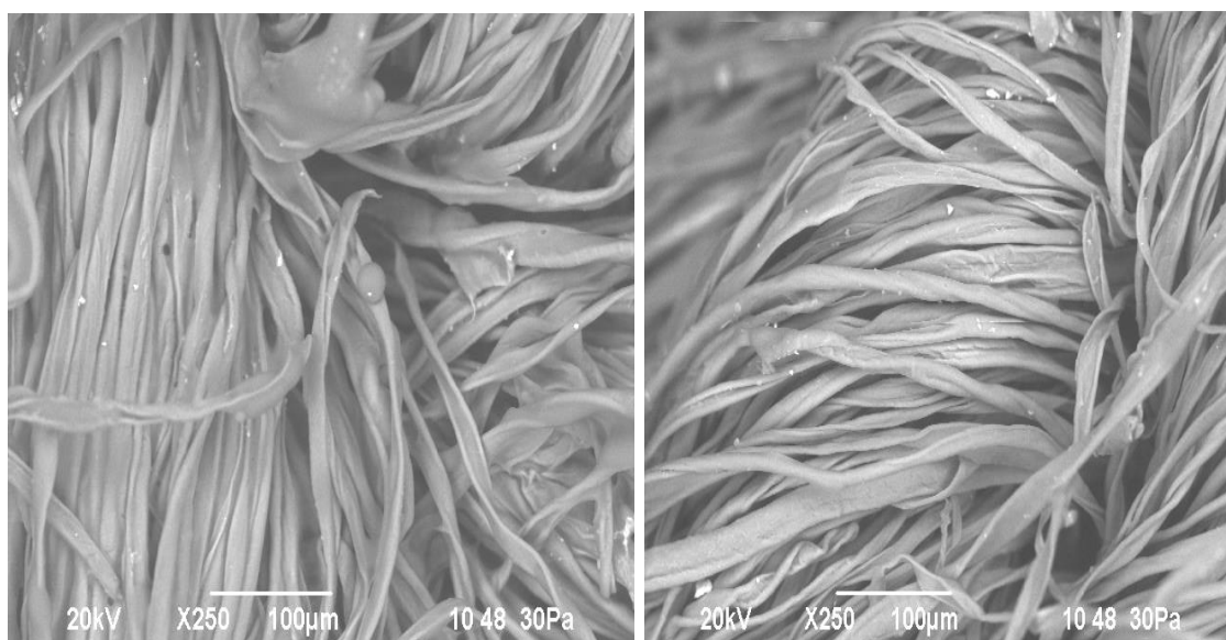
Рисунок 4.12 - Морфология изнаночной (слева) и лицевой (справа) поверхности образца №4
