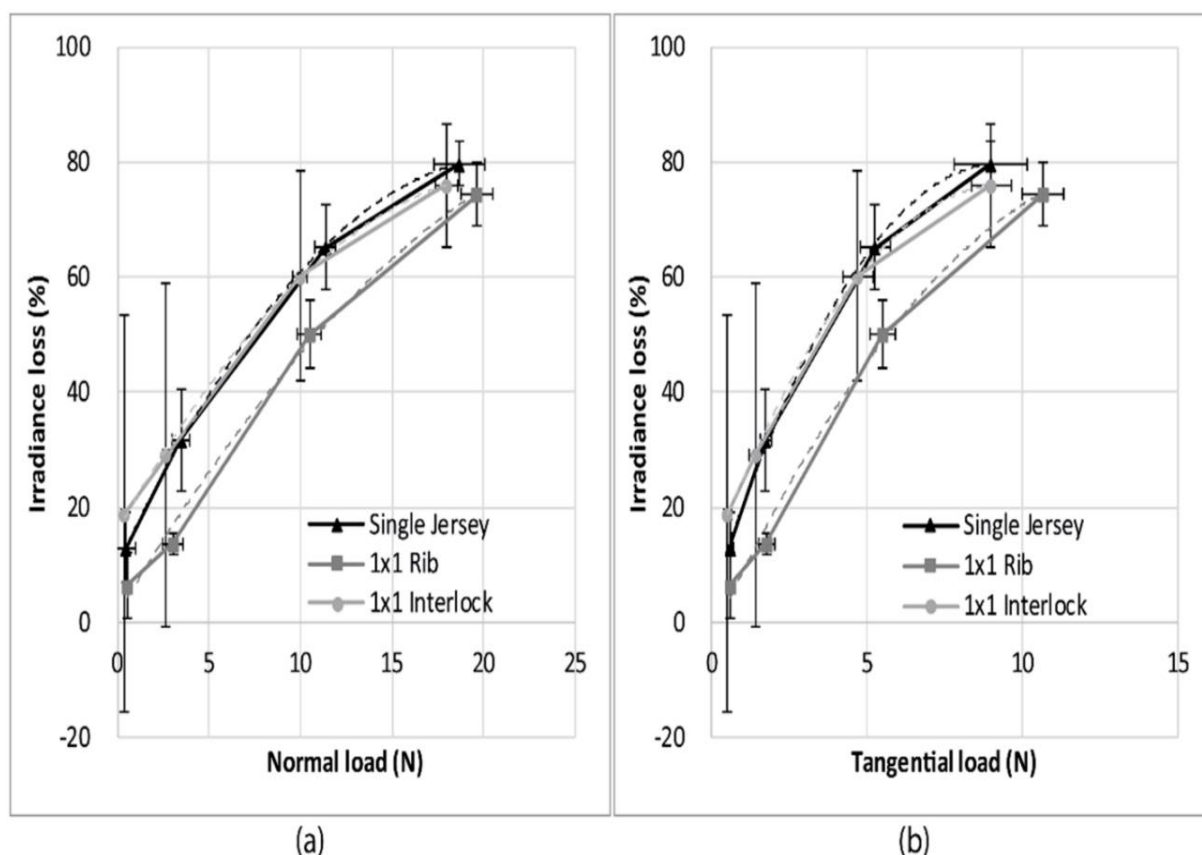
Рисунок 3.6 - Столбики погрешностей показывают стандартное отклонение как потери излучения для трех трикотажных изделий, измененные в зависимости от (a) приложенной нормальной нагрузки и (b) тангенциальной нагрузки.
