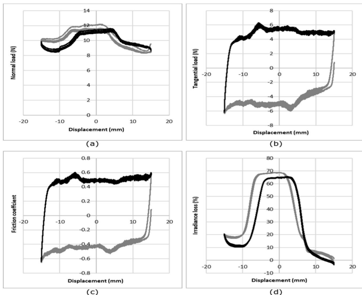
Рисунок 3.5 Эволюция нормальной нагрузки, тангенциальной нагрузки, коэффициента трения и потери освещенности одинарного трикотажного изделия в зависимости от смещения при условной нагрузке 10 Н. Циклы движения ползунка вперед и назад показаны серыми и черными линиями. соответственно. На каждой кривой представлено среднее значение 25 измерений.
