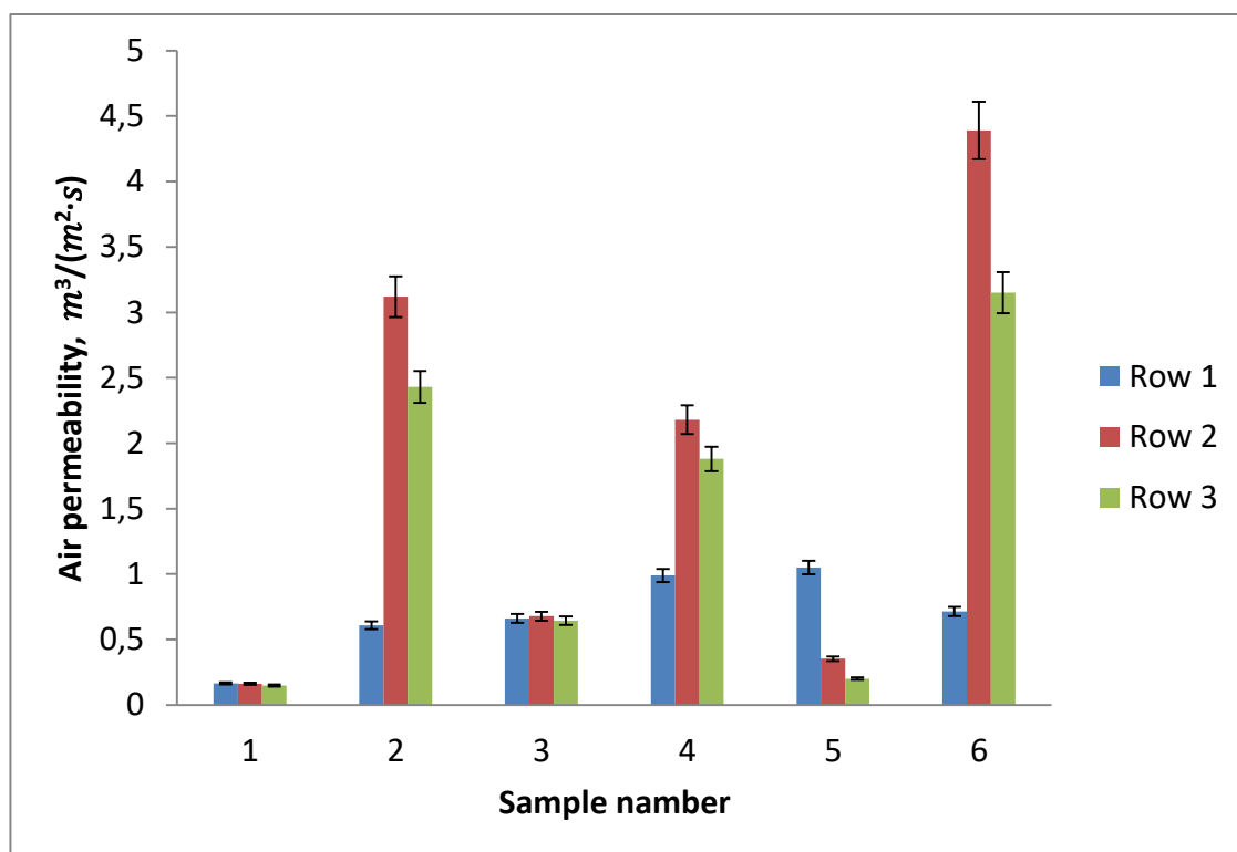
Рисунок 4.3 - Зависимость воздухопроницаемости (А) и паропроницаемости (Б) мембранных материалов от вида текстильного полотна (номер образца и вид полотна по таблице 2.1) и количества слоев полимера: без полимера (Row 1), два слоя (Row 2) и четыре слоя (Row 3) полимера.
