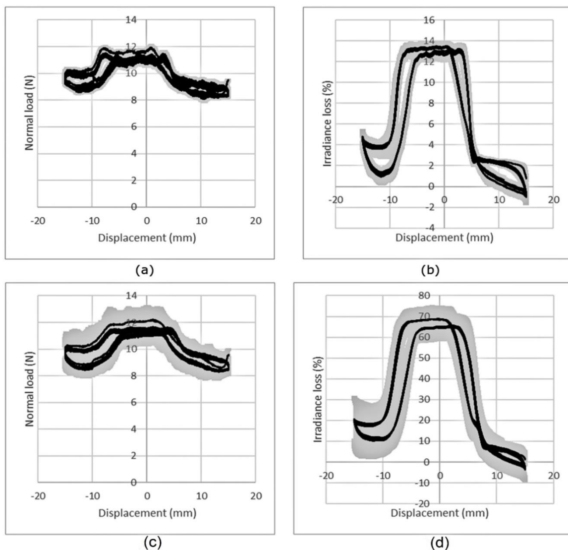
Рисунок 3.4 - Повторяемость и воспроизводимость измерения. Средняя кривая показана черной линией, а стандартное отклонение показано серой областью.
