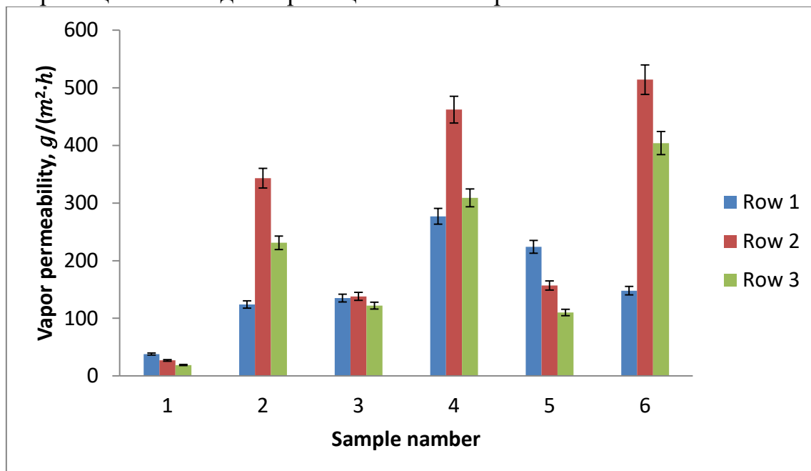
Рисунок 4.4 - Зависимость паропроницаемости мембранных материалов от вида текстильного полотна (номер образца и вид полотна по таблице 2.1) и количества слоев полимера: без полимера (Row 1), два слоя (Row 2) и четыре слоя (Row 3) полимера.
