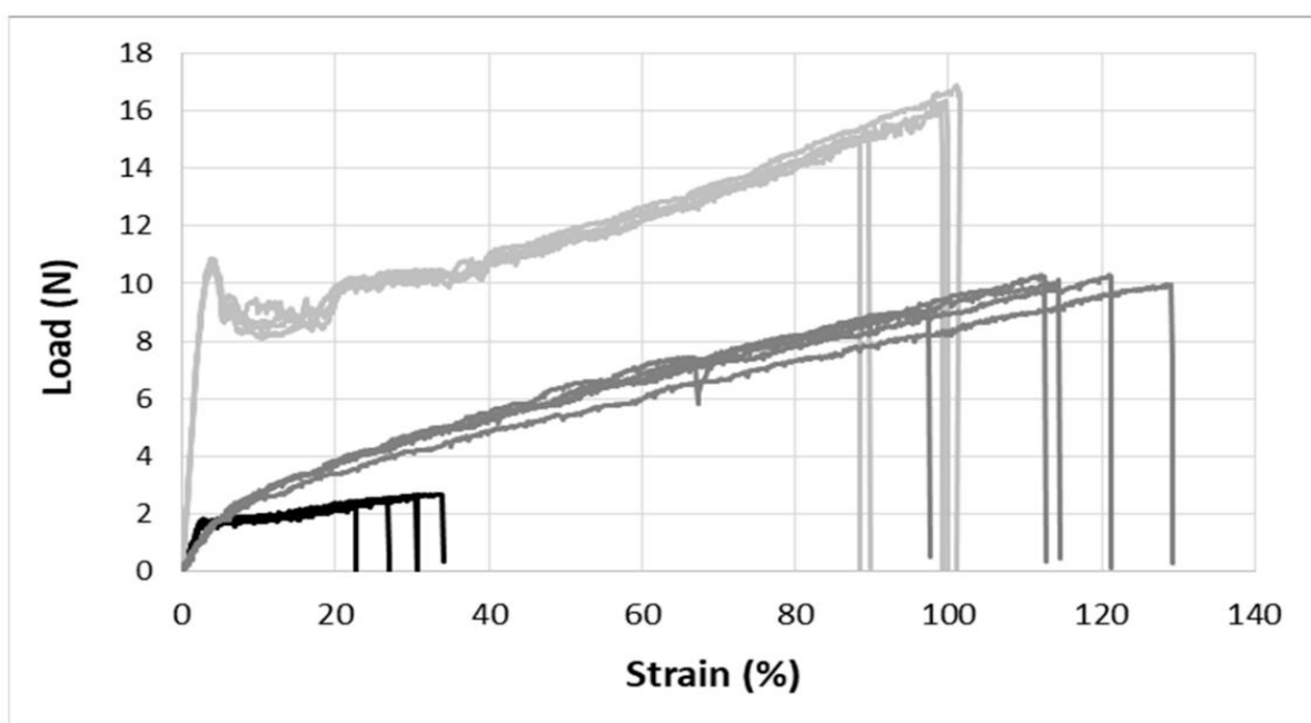
Рисунок 3.1 - Кривая нагрузки-деформации: ПОВ 1 (мягко-серый); ПОВ 2 (черный); ПОВ 3 (темно-серый).
