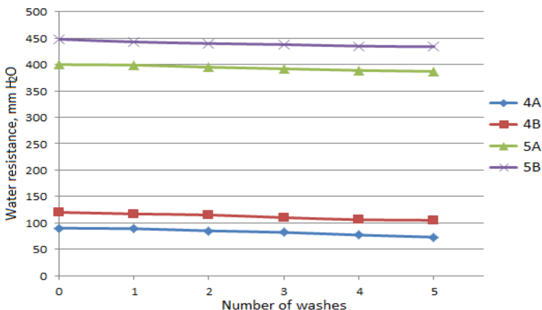
Рисунок 4.17 - Зависимость водоупорности образцов полимерно-текстильных материалов №4 и №5 от числа стирок
