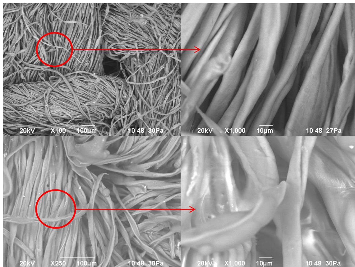
Рисунок 4.9 - СЭМ изображения безворсовой изнаночной стороны махровой хлопковой ткани до нанесения (сверху) и после нанесения акриловой эмульсии (снизу)
