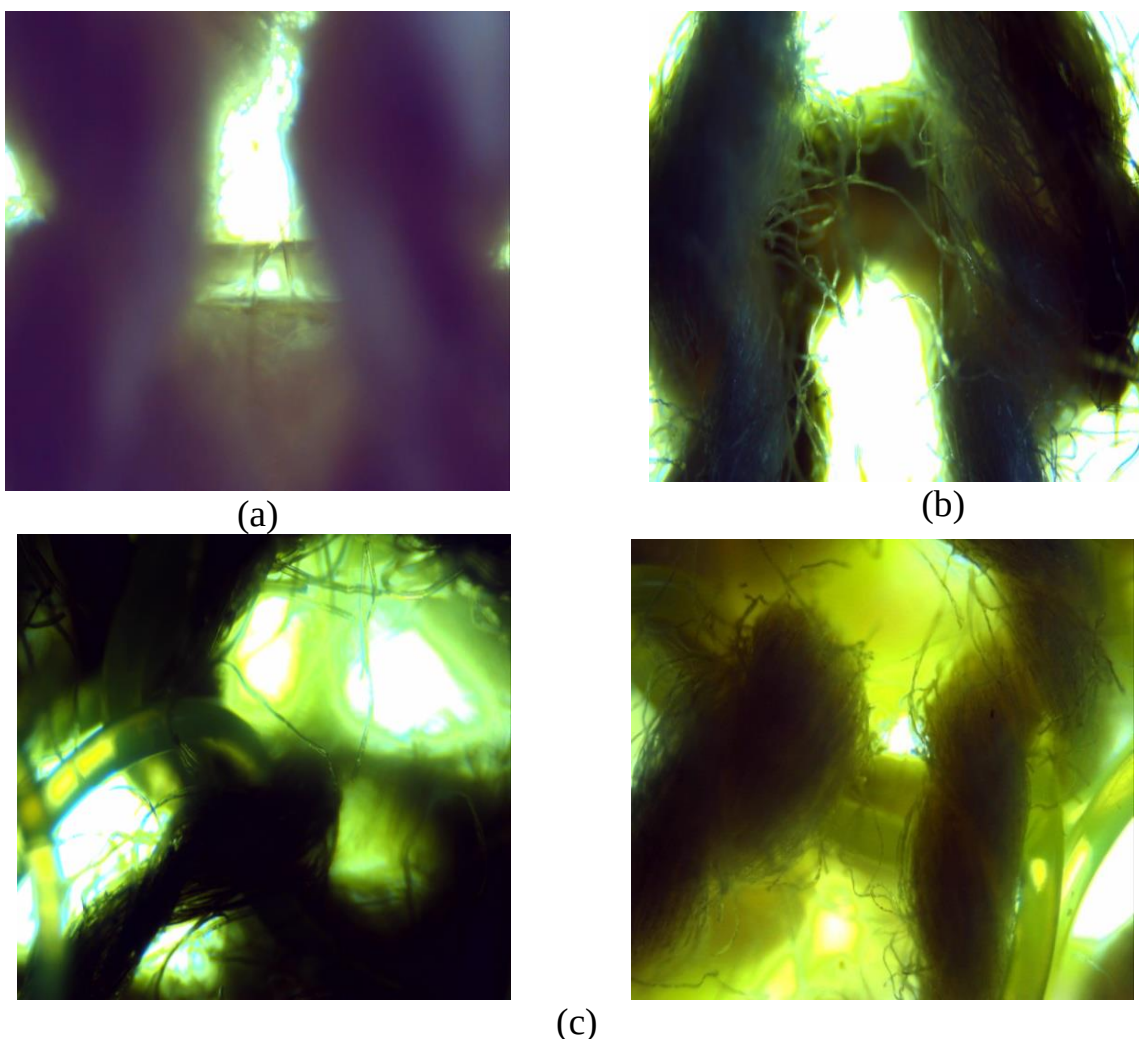
Рисунок 3.8 - Увеличенные изображения полотен: (а) простое переплетение с оптическим волокном в качестве уточной нити; (б) оптическое волокно участвует в простом переплетении; (с) оптическое волокно участвует в плющевом переплетении.
