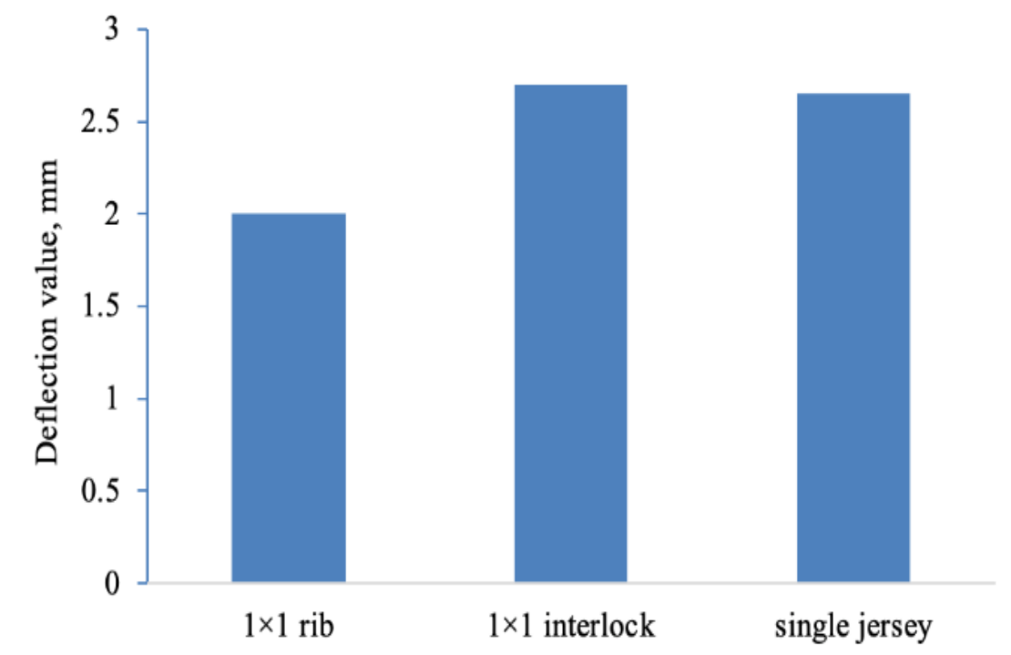
Рисунок 3.7 - Значения отклонения трех тканей для ПОВ в задней части ползунка.
