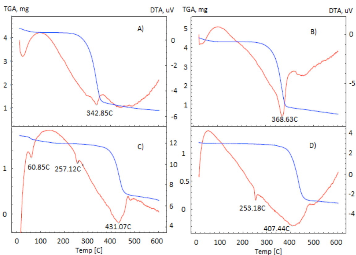
Рисунок 4.7. Кривые ТГА (синяя) и ДТА (красная): х/б ткань (А), х/б ткань-ПМА (Б), полиэфирная ткань (С) и «полиэфирная ткань-ПМА» (Д)
