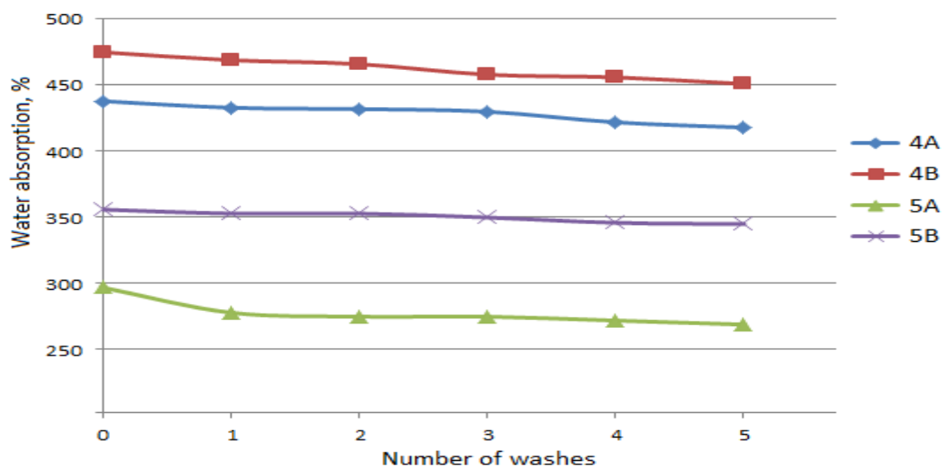
Рисунок 4.16 - Зависимость водопоглощения образцов полимерно-текстильных материалов №4 и №5 от числа стирок
