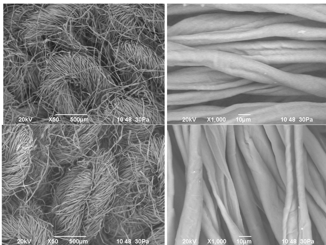
Рисунок 4.10 - СЭМ изображения ворсовой внутренней стороны махровой хлопковой ткани до нанесения (сверху) и после нанесения акриловой эмульсии (снизу)
