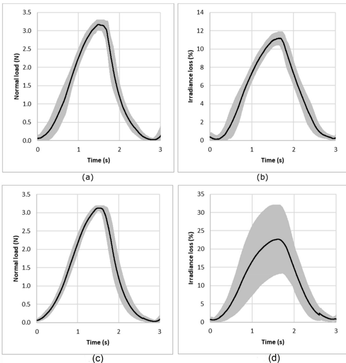
Рисунок 3.2 - Повторяемость и воспроизводимость измерения. Средняя кривая показана черной линией, а стандартное отклонение показано серой областью.
