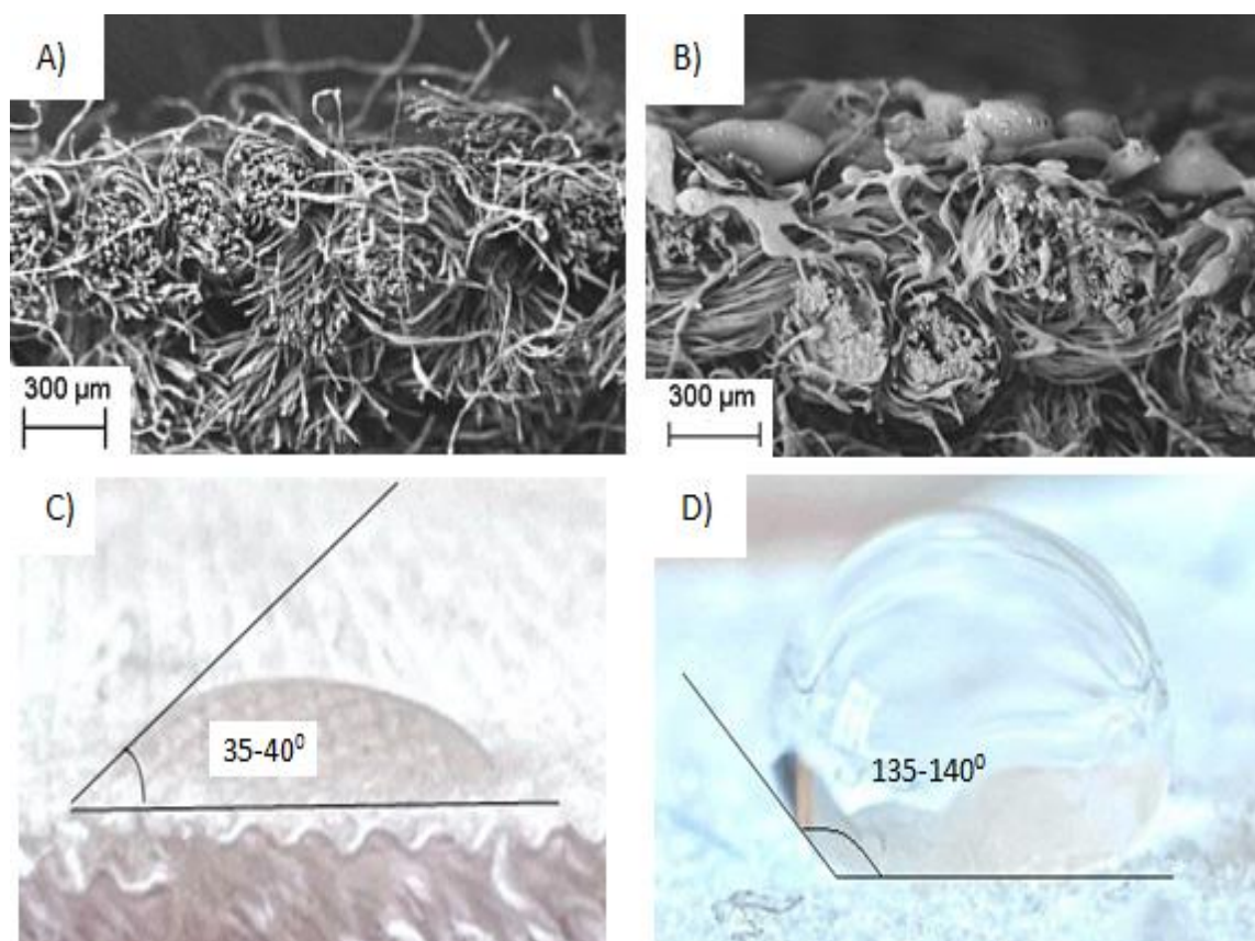
Рисунок 4.5 - Изнаночная поверхность махровой ткани без полимерного слоя (А), с полимерной слоем (В) и капля воды на поверхности без полимера (С), с полимером (D)
