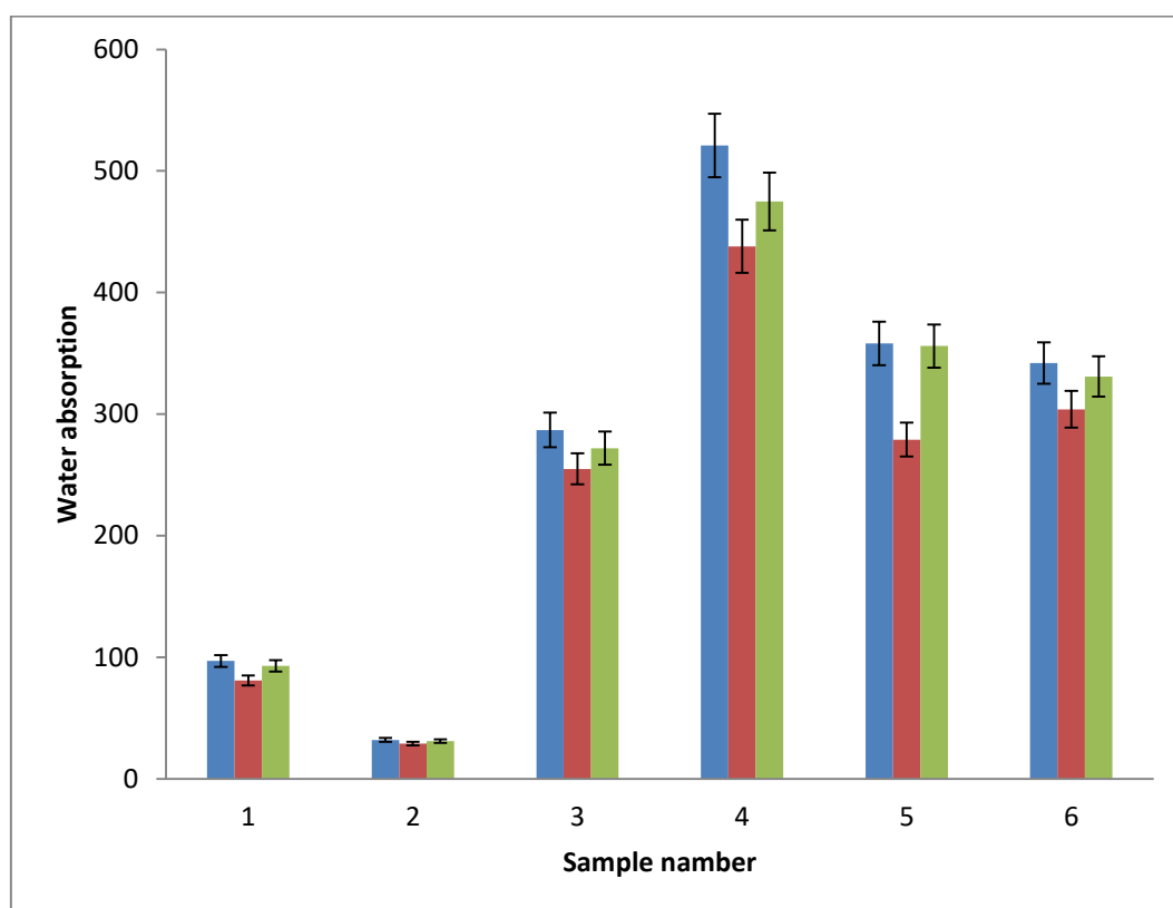
Рисунок 4.1 - Зависимость водопоглощения мембранных материалов от вида текстильного полотна (номер образца и вид полотна по таблице 2.1) и количества слоев полимера: без полимера (1 столбик, синий), два слоя (2 столбик, красный) и четыре слоя (третий столбик, зеленый) полимера
