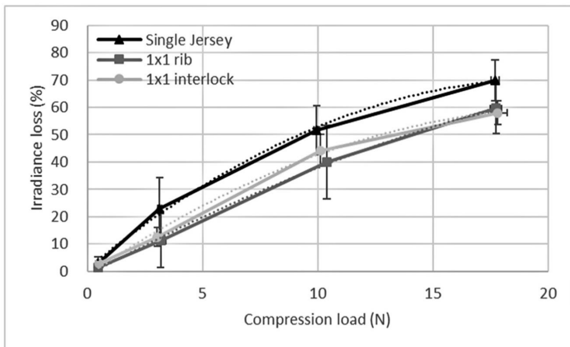
Рисунок 3.3 - Эволюция потери излучения в зависимости от приложенной силы сжатия, при этом столбики погрешностей обозначают стандартное отклонение. Аппроксимационные кривые второго порядка показаны пунктирными линиями.
