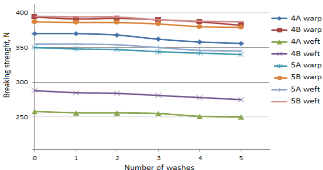
Рисунок 4.14 - Зависимость разрывной силы образцов полимерно-текстильных материалов №4 и №5 от числа стирок
