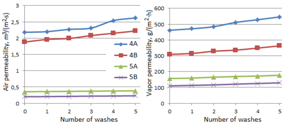
Рисунок 4.18 - Зависимость воздухопроницаемости (слева) и паропроницаемости (справа) образцов полимерно-текстильных материалов №4 и №5 от числа стирок
