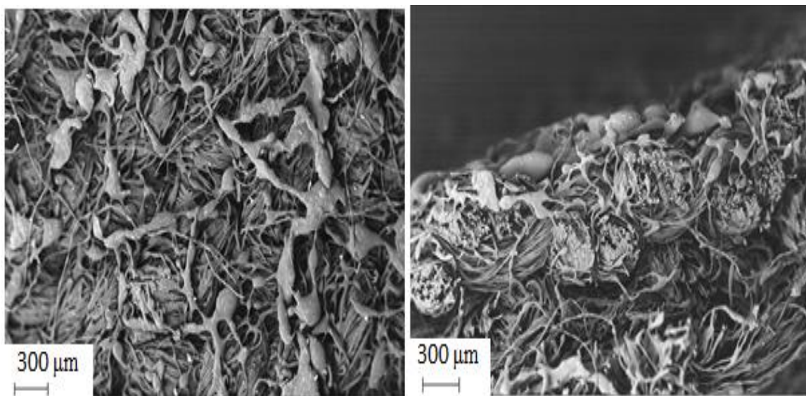
Рисунок 4.13 - Морфология полимерного слоя на поверхности (слева) и на поперечном сечении образца №5
