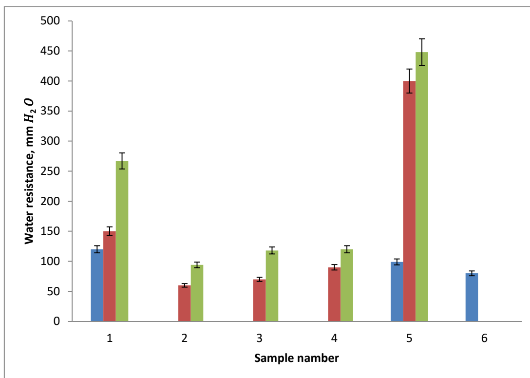
Рисунок 4.2 - Зависимость водоупорности мембранных материалов от вида текстильного полотна (номер образца и вид полотна по таблице 2.1) и количества слоев полимера: без полимера (1 столбик, синий), два слоя (2 столбик, красный) и четыре слоя (третий столбик, зеленый) полимера
