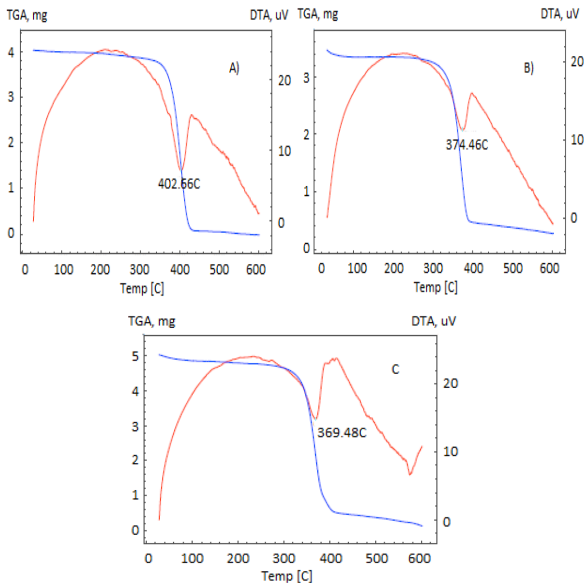
Рисунок 4.6. Кривые ТГА (синяя) и ДТА (красная) ПМА (А), махровой х/б ткани (В) и мембранного материала «Махровая ткань-ПМА» (С)
