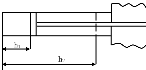
Сурет 3 - Газ қозғалмалы поршені
