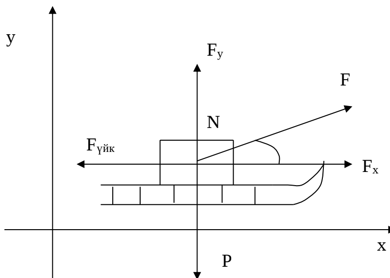
Сурет 1 - Жүк тиелген шананың горизонталь бетпен қозғалысы
