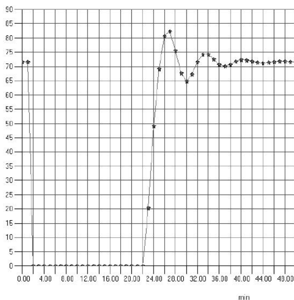
Сурет 6. Колоннаның қыздырғышындағы деңгейді автоматты басқару жүйесінің графигі
