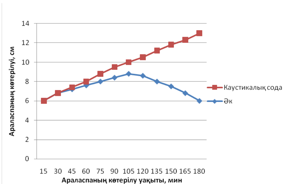
Сурет 1. Уақыт бойынша газ-бетон қоспасының өсу кестесі
