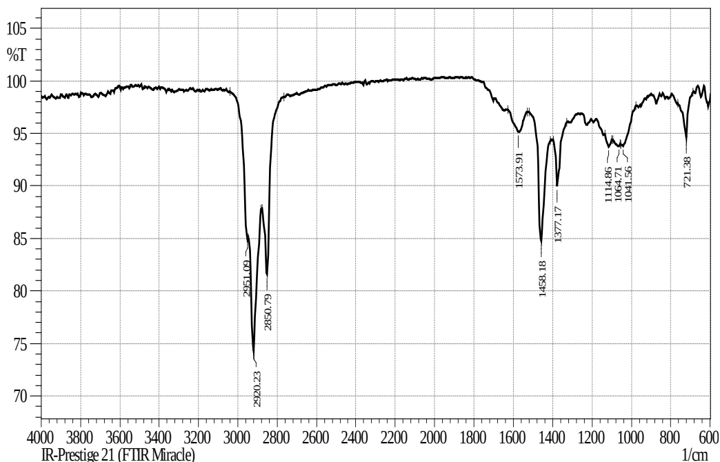
Рис. 1 – ИК-спектры
