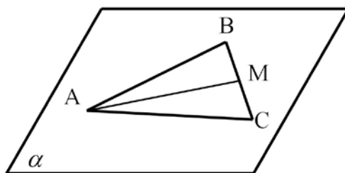
2-сурет. \alpha жазықтығында ABC үшбұрышы
