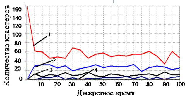
Рис. 3. Временная история количества кластеров от различных порядков для w = 8 , таблица 4X40. Эксперимент для случая АОД. Порядки кластеров: 1-й, 2-й, 3-й, 4-й
