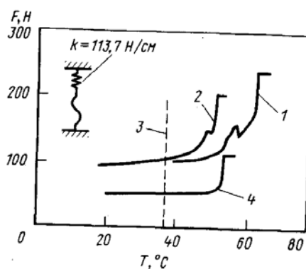
Рис. 2. Изменение температуры начала и конца аустенитной точки образца.
