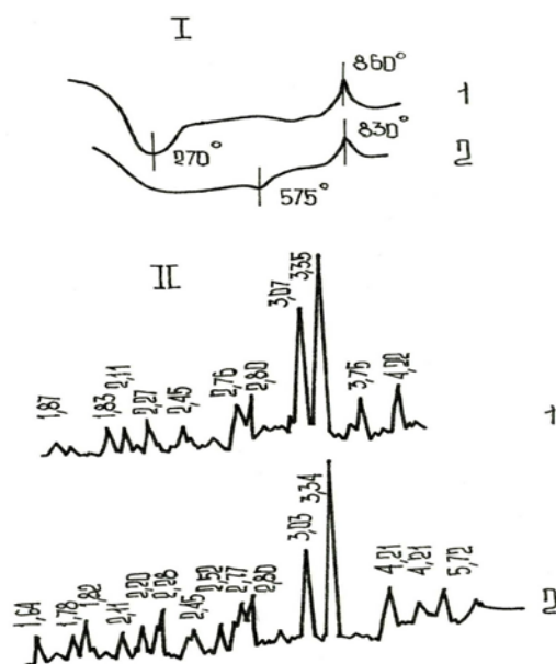
Сурет 2. Түрлі құрамдағы цемент және кремнеземдік материалдар негізіндегі автоклавталған үлгілердің термограммалары мен рентгенограммалары: 1 - цемент қоспасынан және аз қайнатылатын шикізатты қайта өңдеу қалдықтарынан жасалған үлгілер; 2 - цемент және кварц құм қоспасы үлгілері
