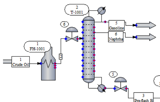
Сурет 5. Ректификациялық қондырғылардың реттелетін тізбектері
