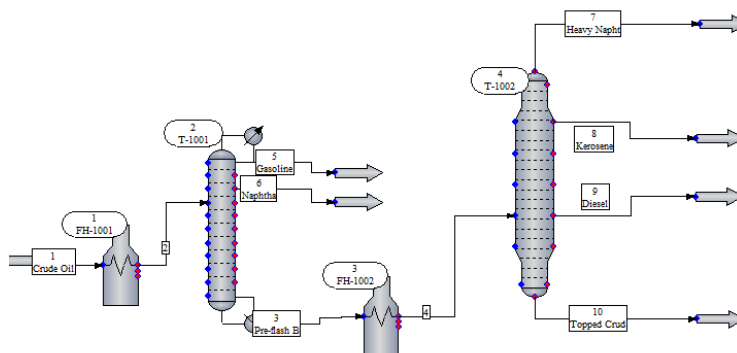
Сурет 2. ChemCad-тағы технологиялық сұлбаның бейнесі
