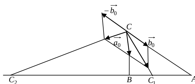
Рис.1 - Треугольник ABC
