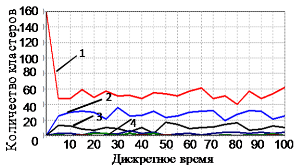
Рис. 2. Временная история количества кластеров от различных порядков для w = 2 , таблица 4X40. Эксперимент для случая АОД. Порядки кластеров: 1-й, 2-й, 3-й, 4-й
