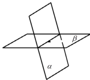
1-сурет. Аксиома жазықтығы
