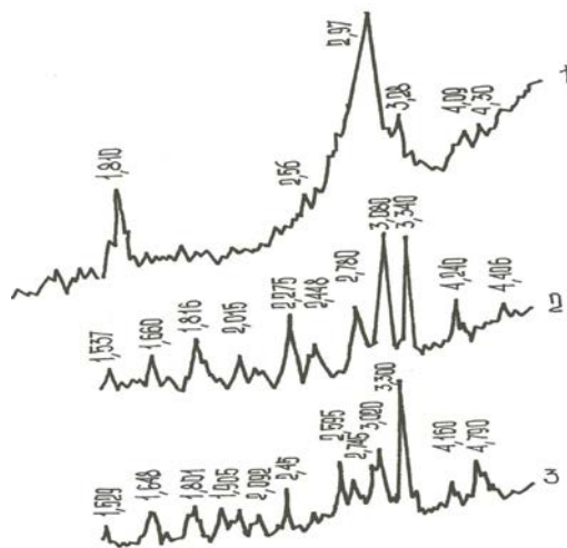
Сурет 1. Қоспалары бар әк-кварц үлгілерінің рентгенограммалары: 1 - 3% \text{Na}_2\text{O} әк және кварц қоспасы бар үлгілер; 2 - 9% \text{Al}_2\text{O}_3 әк және кварц қоспасы бар үлгілер; 3 - 3% \text{Na}_2\text{O} және 9% \text{Al}_2\text{O}_3 әк және кварц қоспасы бар үлгілер.
