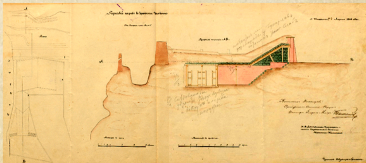
Сурет №2 – План и профиль порохового погреба крепости Чимкент. г. Ташкент. 24 апреля 1866 г. [1].
