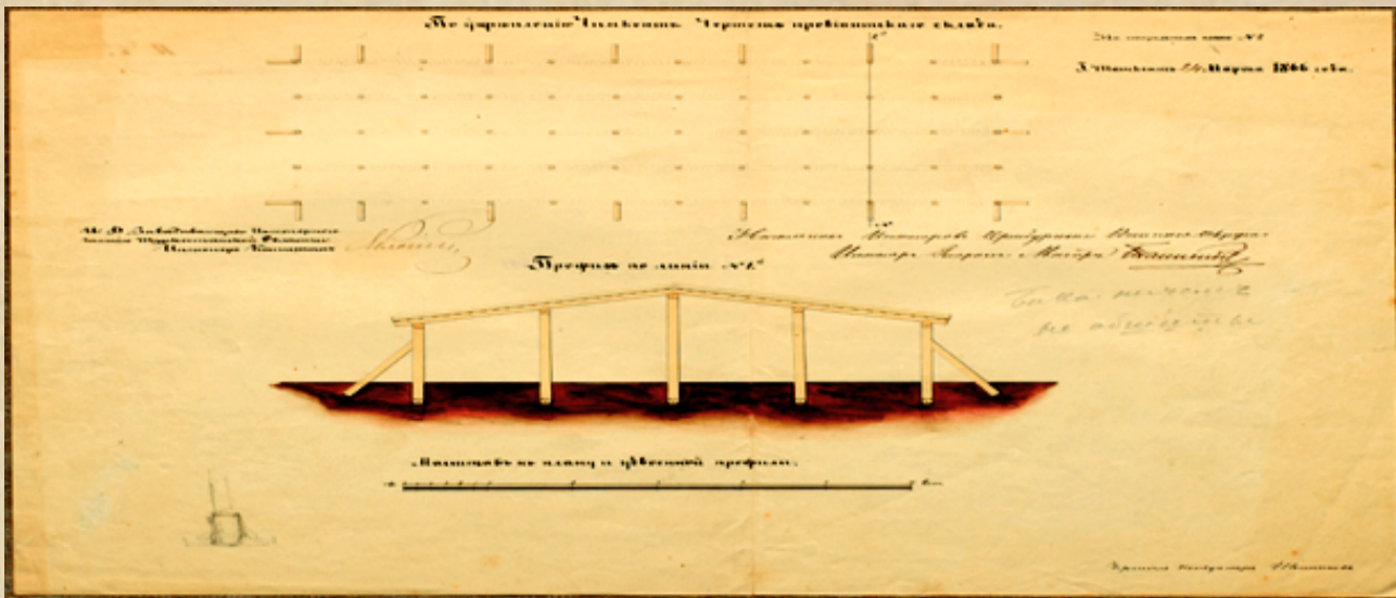
Сурет №3 – По укреплению крепости Чимкент. Чертеж провиантского склада. г. Ташкент. 24 апреля 1866 г. [2].
